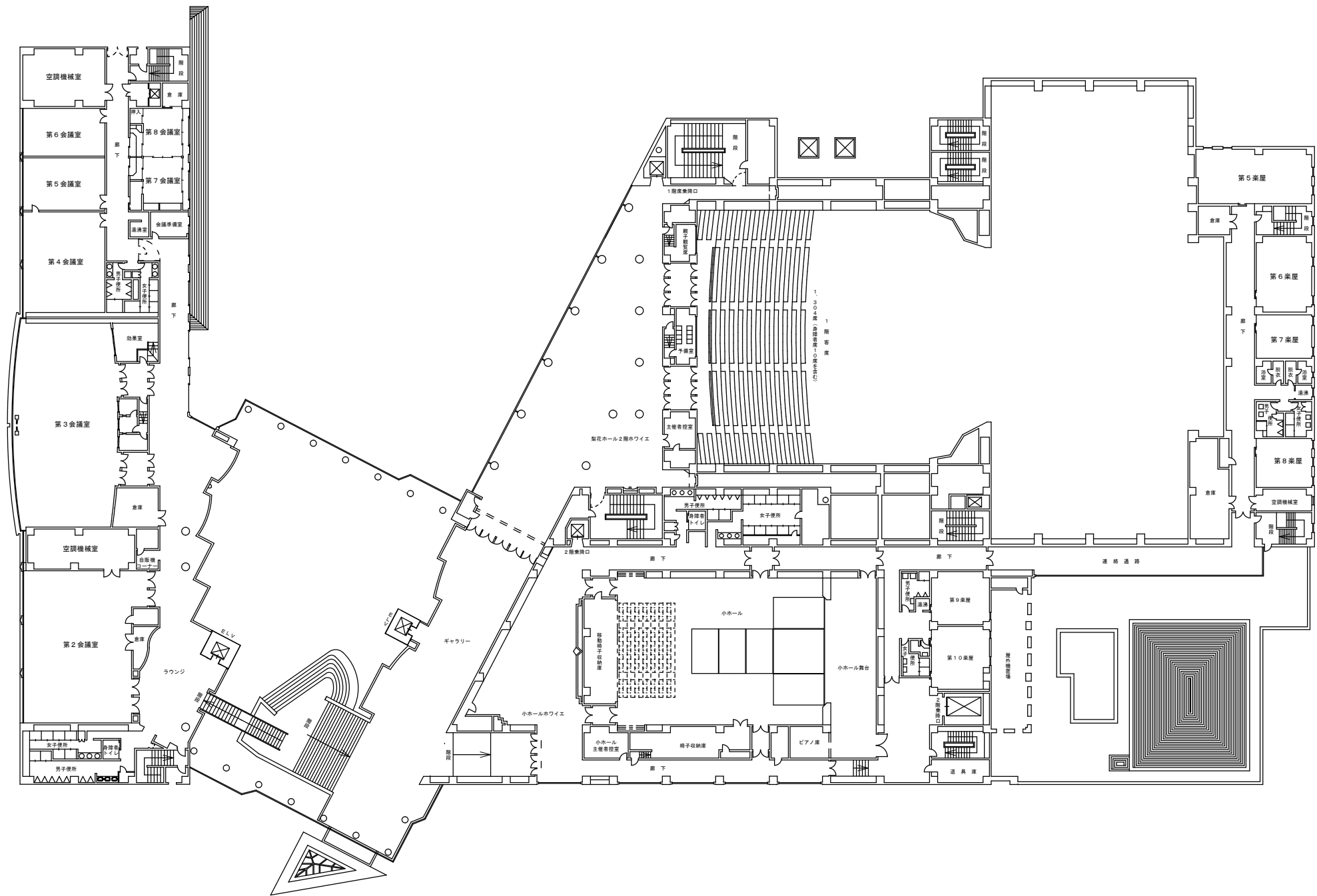
鳥取県立県民文化会館(とりぎん文化会館) 2階平面図
