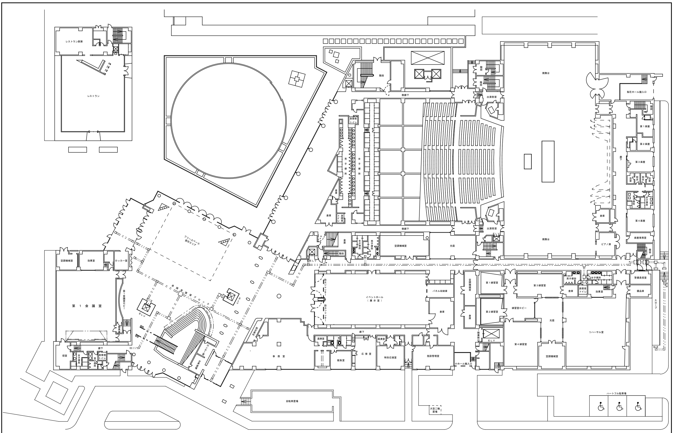
1 階 平 面 図
